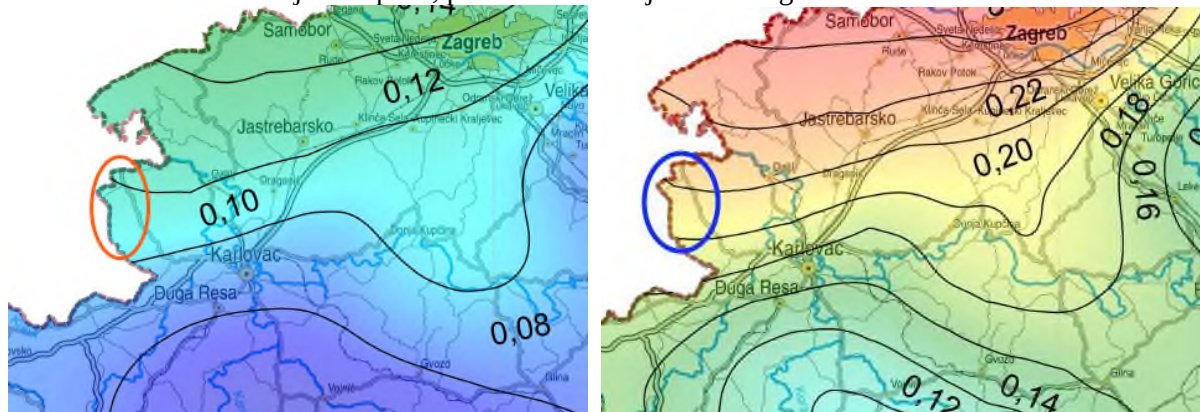
Slike 3 i 4: Zumirani Izvodi iz Karte potresnih područja RH za općinu Žakanje i kontaktno područje; Poredbeno vršno ubrzanje tla tipa A, povratno razdoblje 95 i 475 godina
