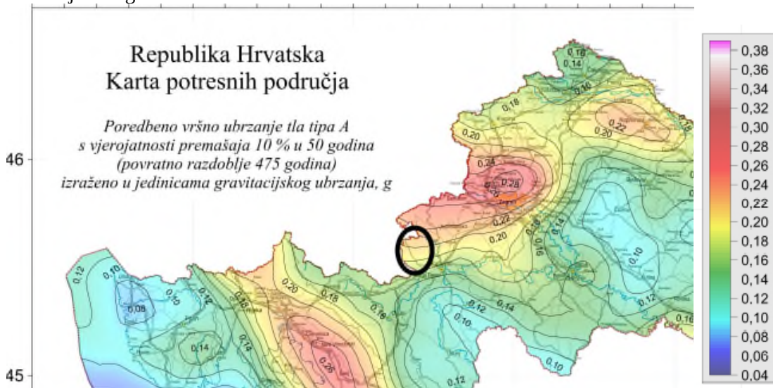
Slika 2: Izvod iz Karte potresnih područja u RH; Poredbeno vršno ubrzanje tla tipa A, povratno razdoblje 475 godina
